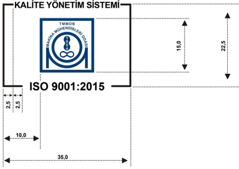
Şekil 1: ISO 9001:2015 ve MMO Logosunun ölçülendirilmesi
